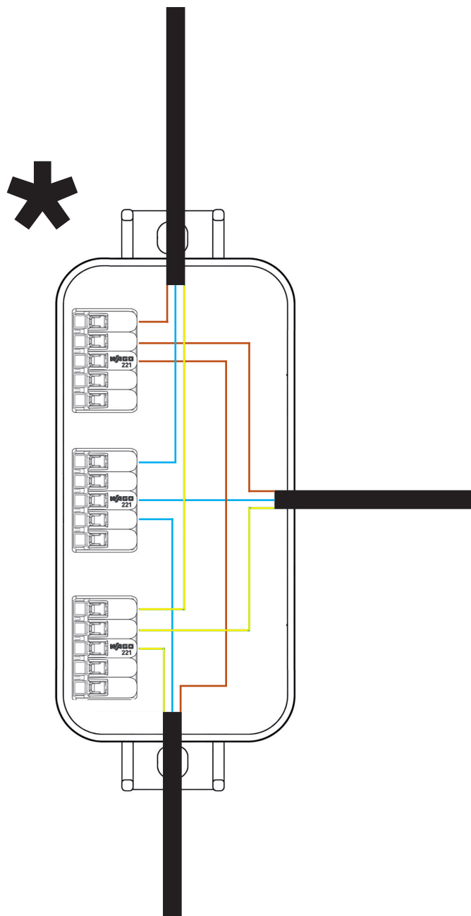
E160_Schema Elektro (Landstrom)
