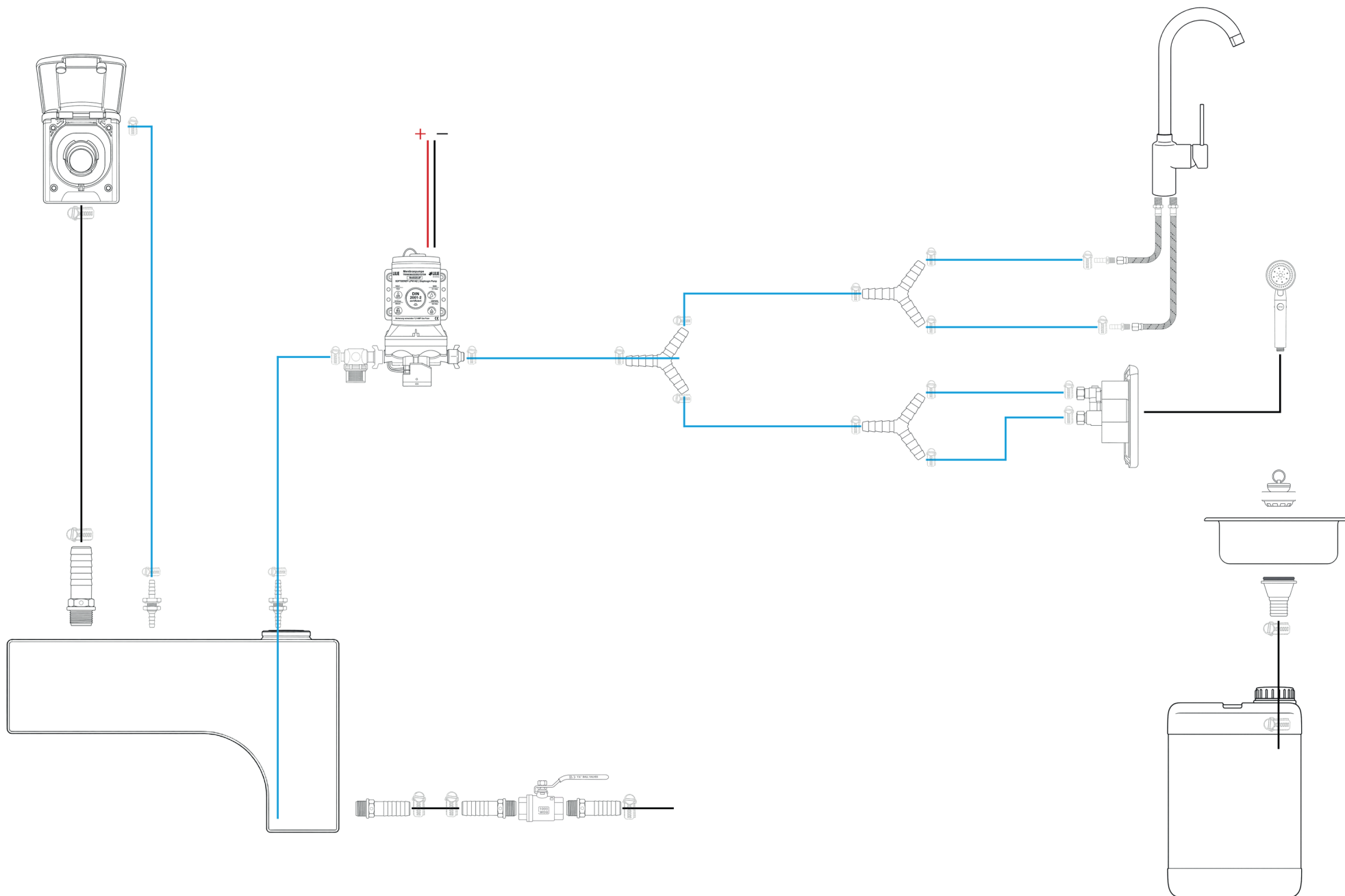
W120_Schema Wasser (ohne Boiler, Abwasserkanister)
