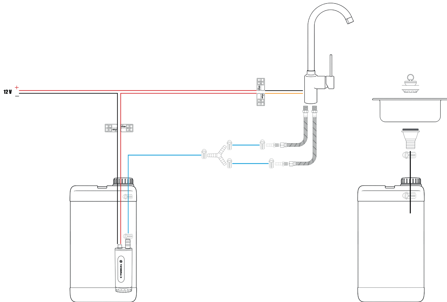
W130_Schema Wasser (Tauchpumpe, Kanister)
