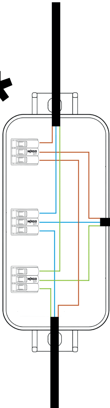
E160_Schema Elektro (Landstrom)
