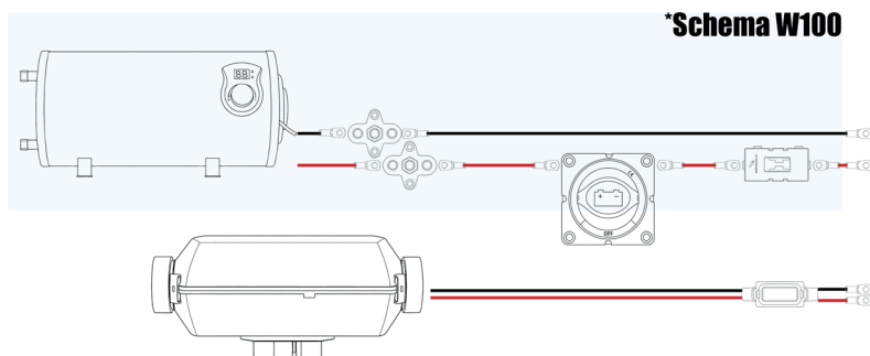
E100_Schema Elektro (Basic)
