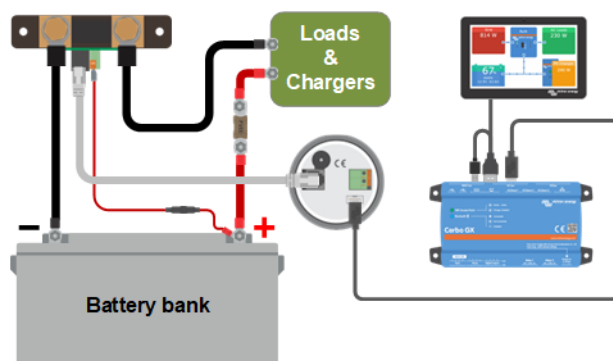
Beispiel für einen Batterieмонitor, der an ein GX-Gerät angeschlossen wird.
